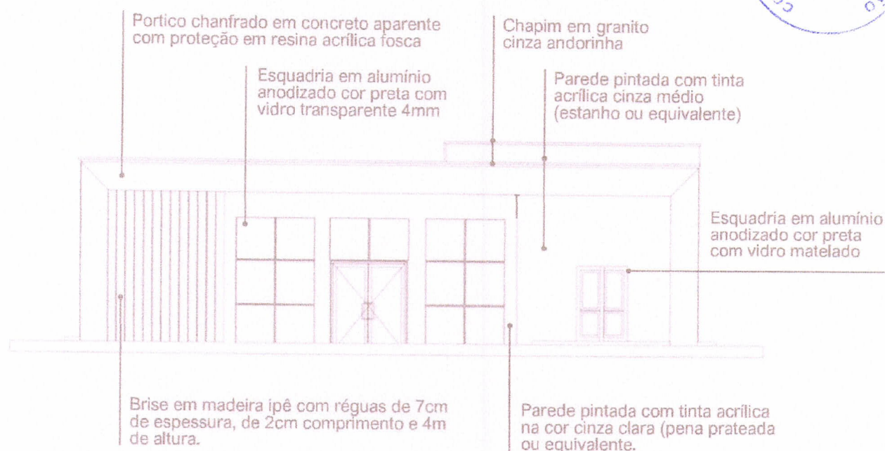
Figura 2 – Fachada 01.
